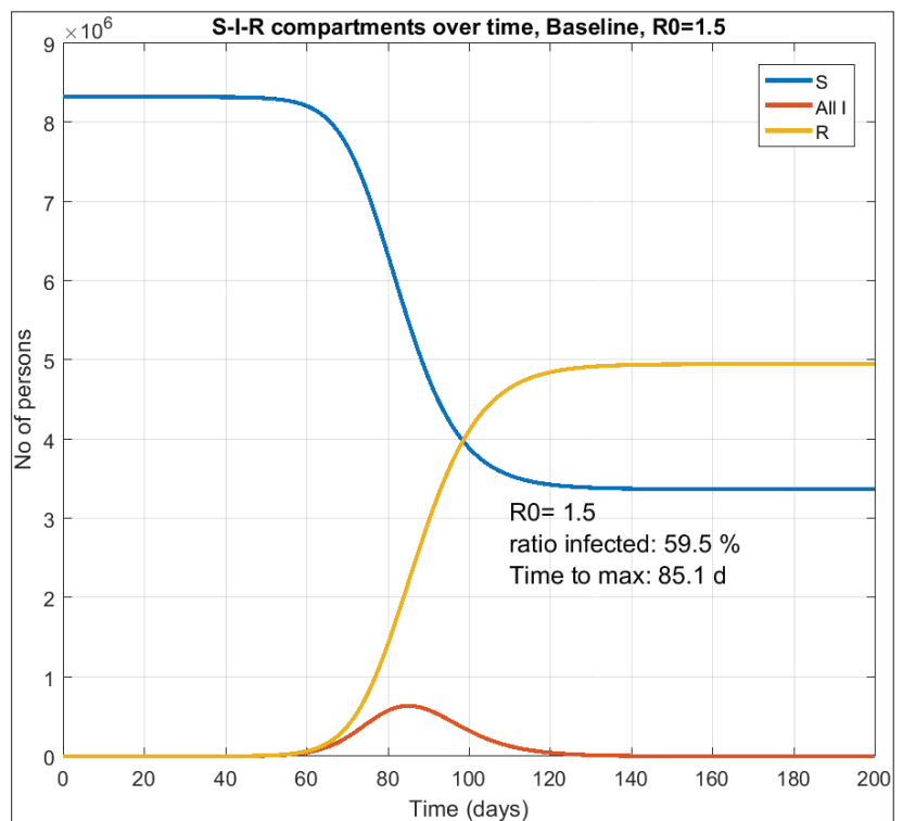
Abbildung 5 Änderung der Reservoirs von S, I, R über den zeitlichen Verlauf. S = Reservoir Ansteckbare (Susceptibles); I = Infizierte (Infectious); R = Gesunde (Recovered). Erklärung s. Text.
